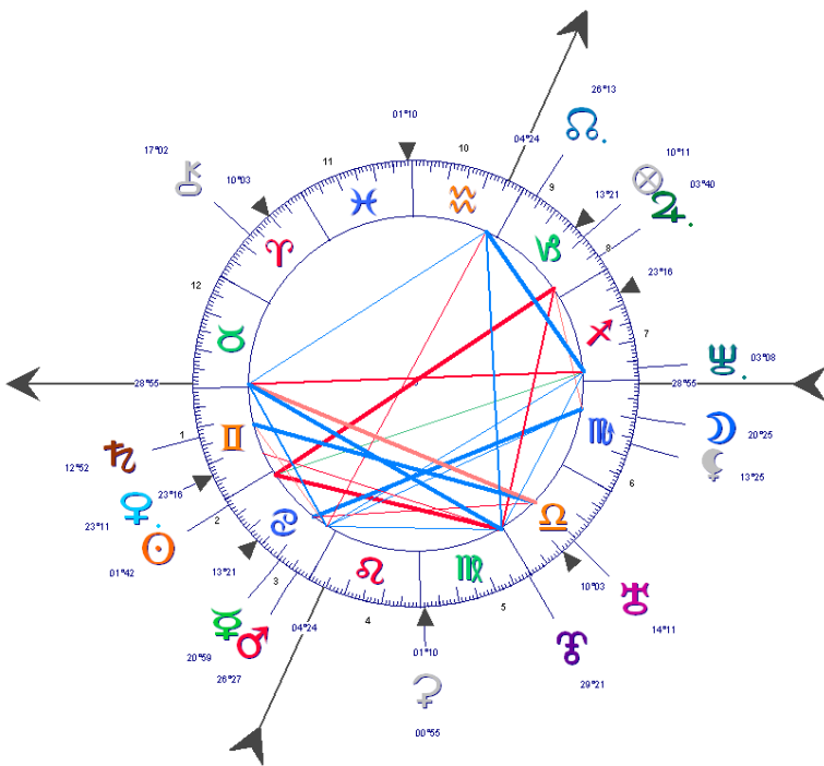
Equivalents déclinaison-longitude
