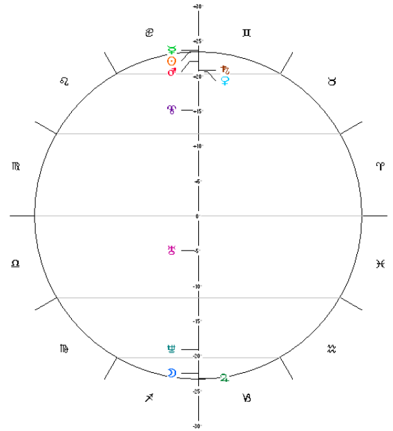
Equivalents déclinaison-longitude
